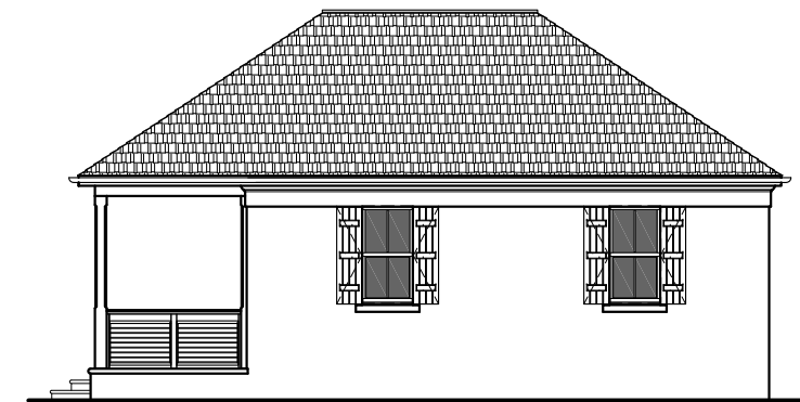
RIGHT ELEVATION
